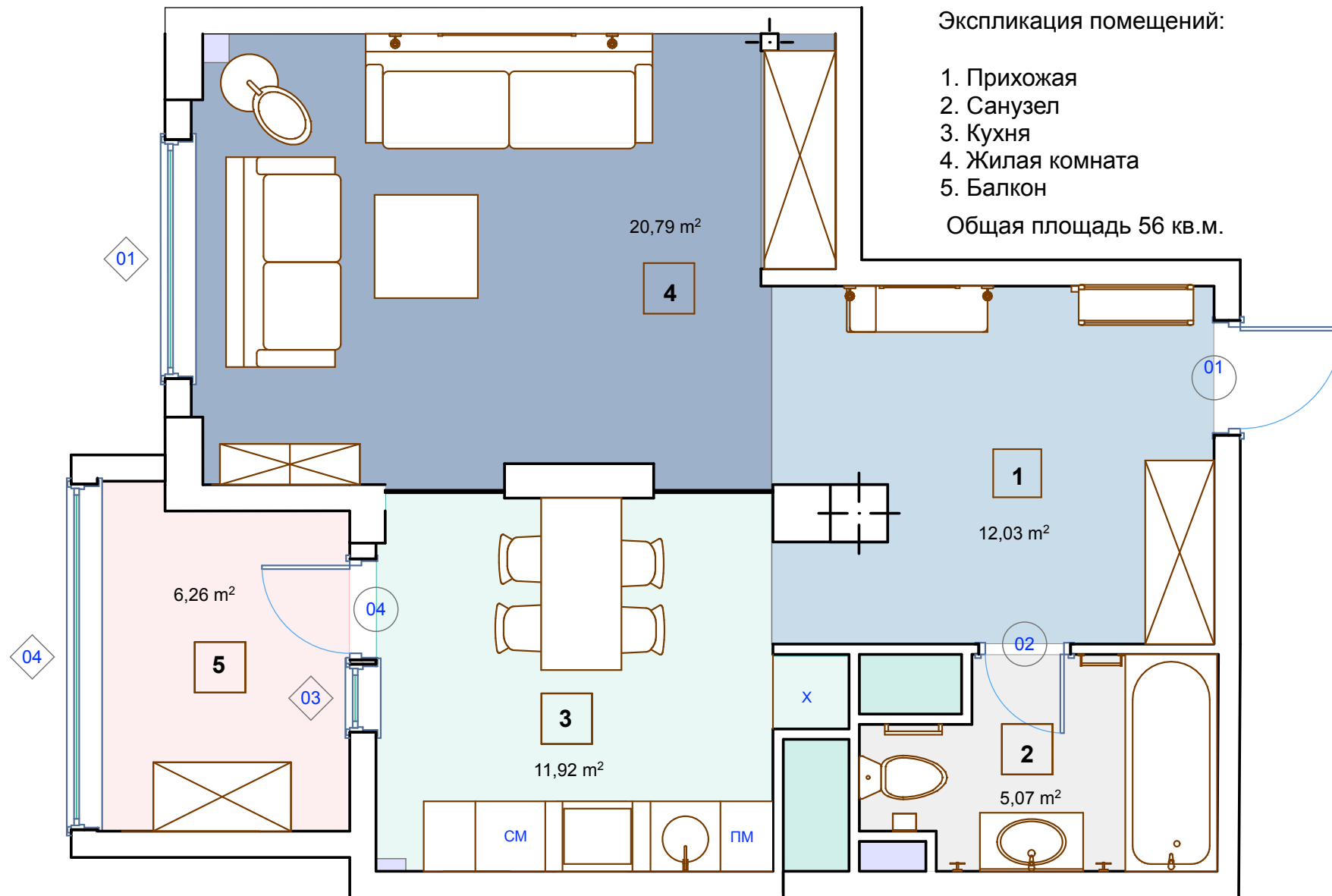
План расстановки мебели и сантехники, М1:50 с экспликацией помещений
